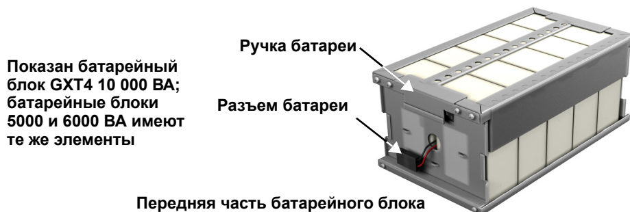
Изображение 4 Встроенный батарейный блок с разъемом
