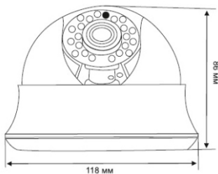
Рис.1 Вид сбоку
