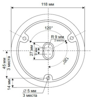
Рис.3 Крепежная платформа
